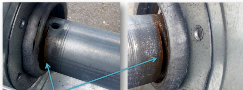
L'axe du rideau est cisailé par le rideau par manque de graissage et de contrôle
